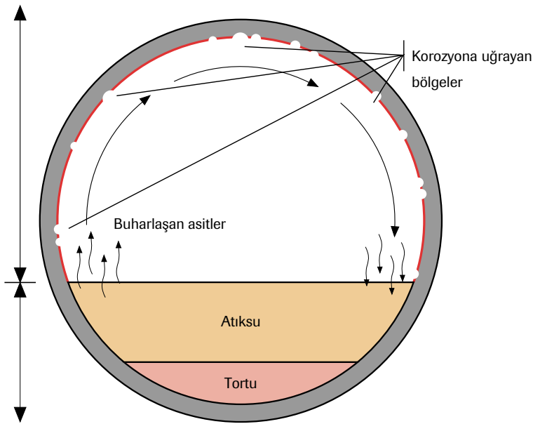
Kimyasal korozyona karşı savunmasız beton borularda aşınmalar meydana gelir.
